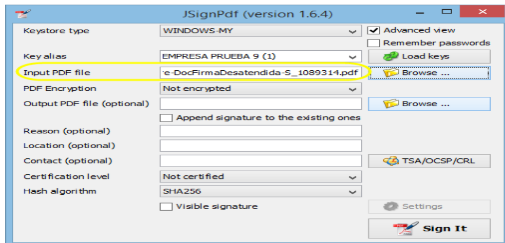
Fig. 3: Input PDF file – ruta de ubicación del archivo PDF a firmar
