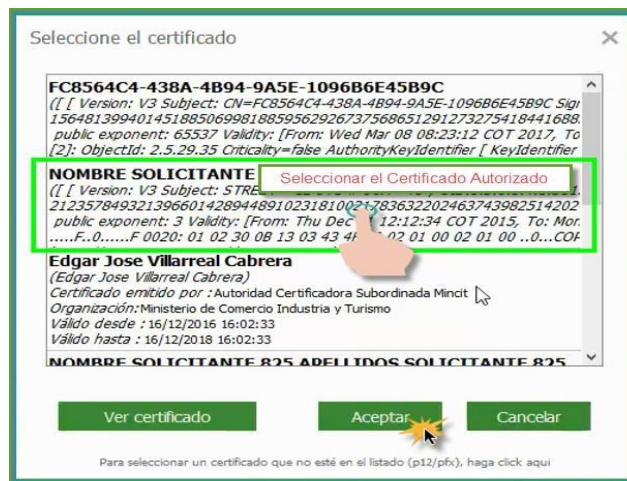
Fig. 12: Certificados instalados
