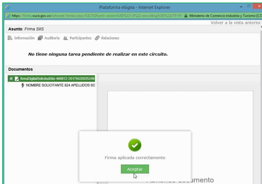
Fig. 15: Firma completada
